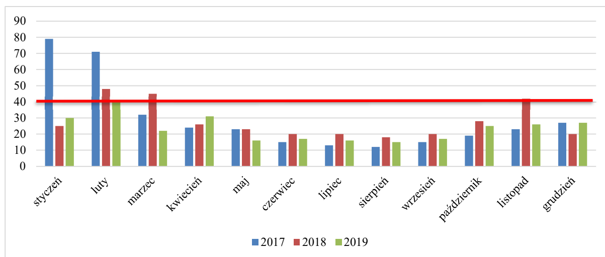
Rysunek 11 Średnie stężenie pyłu PM10 na stacji w Dzierżonowie ul. Piłsudskiego 26 w latach 2017 - 2019 ( \mu\text{g}/\text{m}^3 )
