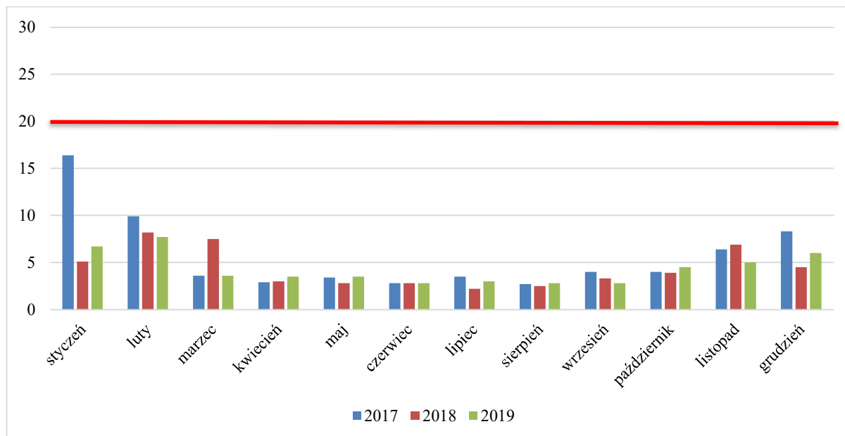
Rysunek 9 Średnie stężenie dwutlenku siarki na stacji w Dzierżoniowie ul. Piłsudskiego 26 w latach 2017 - 2019 (µg/m 3 )
