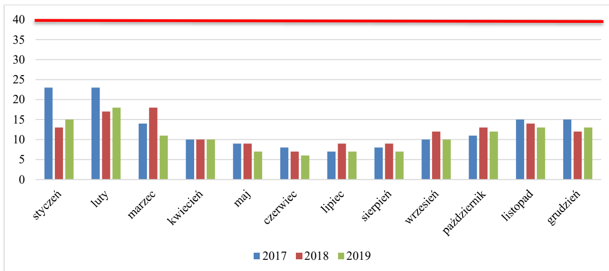
Rysunek 10 Średnie stężenie dwutlenku azotu na stacji w Dzierżonowie ul. Piłsudskiego 26 w latach 2017 - 2019 ( \mu\text{g}/\text{m}^3 )
